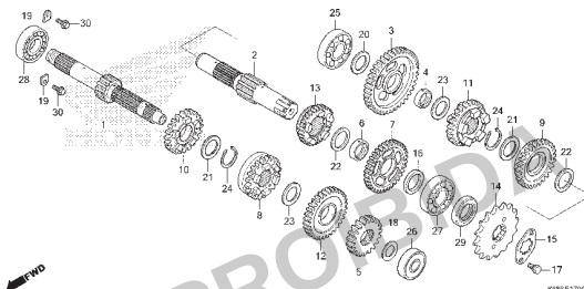
M-17 Transmissão
