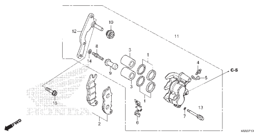
C-17 Cáliber do Freio Traseiro
