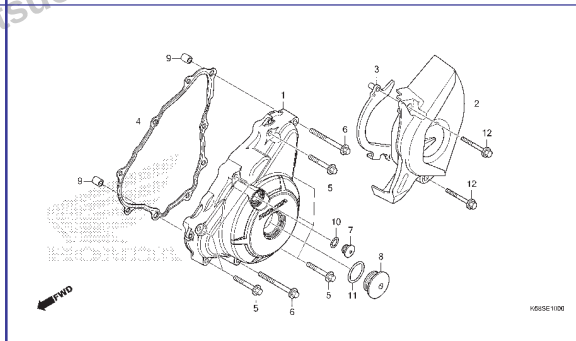
M-10 Tampa Lateral Esquerda
