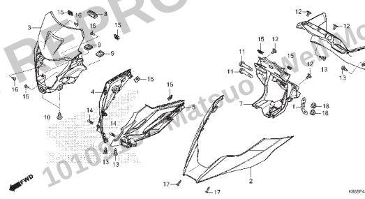
C-43 Para-lama Superior • Defletor Dianteiro
